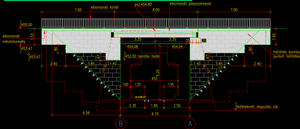
Az eredeti híd oldalnézete
