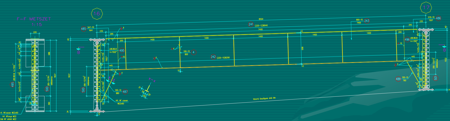
KÖZBENSŐ HOSSZTARTÓ OLDALNÉZET 1:15 készül: 2db
