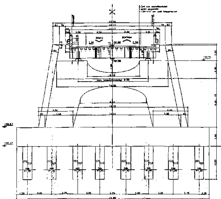
MEDER TÁMASZ (C) KERESZTMETSZET M1:100 (62+848,25 SZ.)
