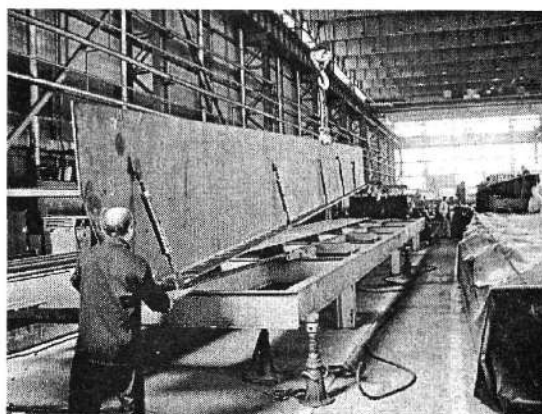
hossztartó gerinc és övlemez előgyártása (6. kép)
