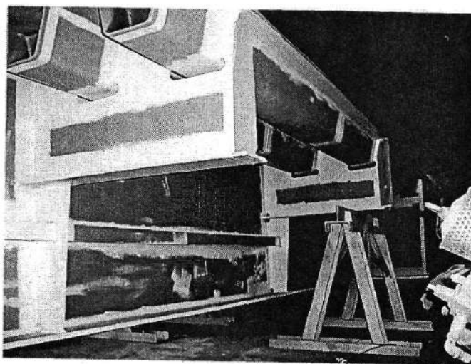
Merevítő tartó gyári felületvédelme (14. kép)
