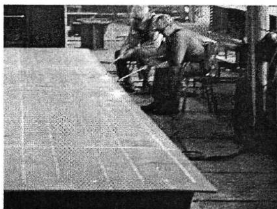
pályaeység egyengetése (5. kép)
