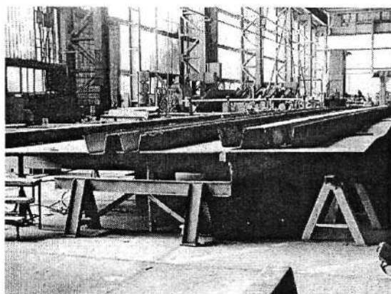
pályalemezre a trapézbordák elhelyezése (3. kép)
