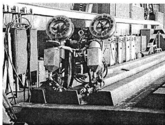
trapézborða nyakvarratok hegesztése kétféjes fedettívű automatával (4. kép)
