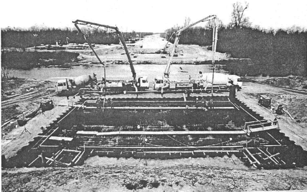
A fejlemez betonozása (2. kép)
