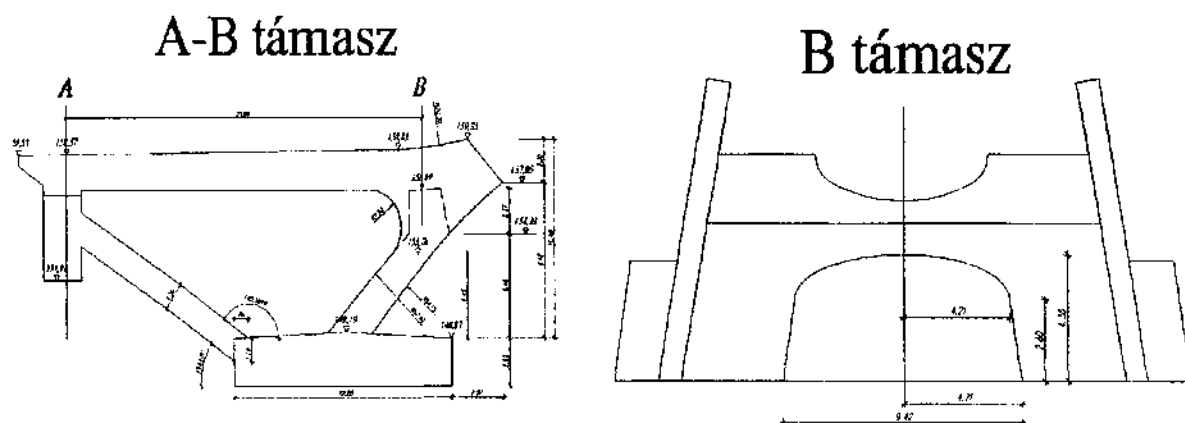
6. sz. ábra (oldalnézet és előlnézet)
