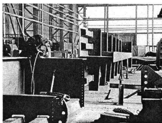
pozícióba forgatva hegesztések elvégzése (8. kép)
