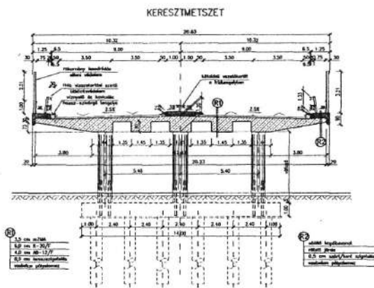
1. ábra: „A” jelű hídág keresztmetszete
