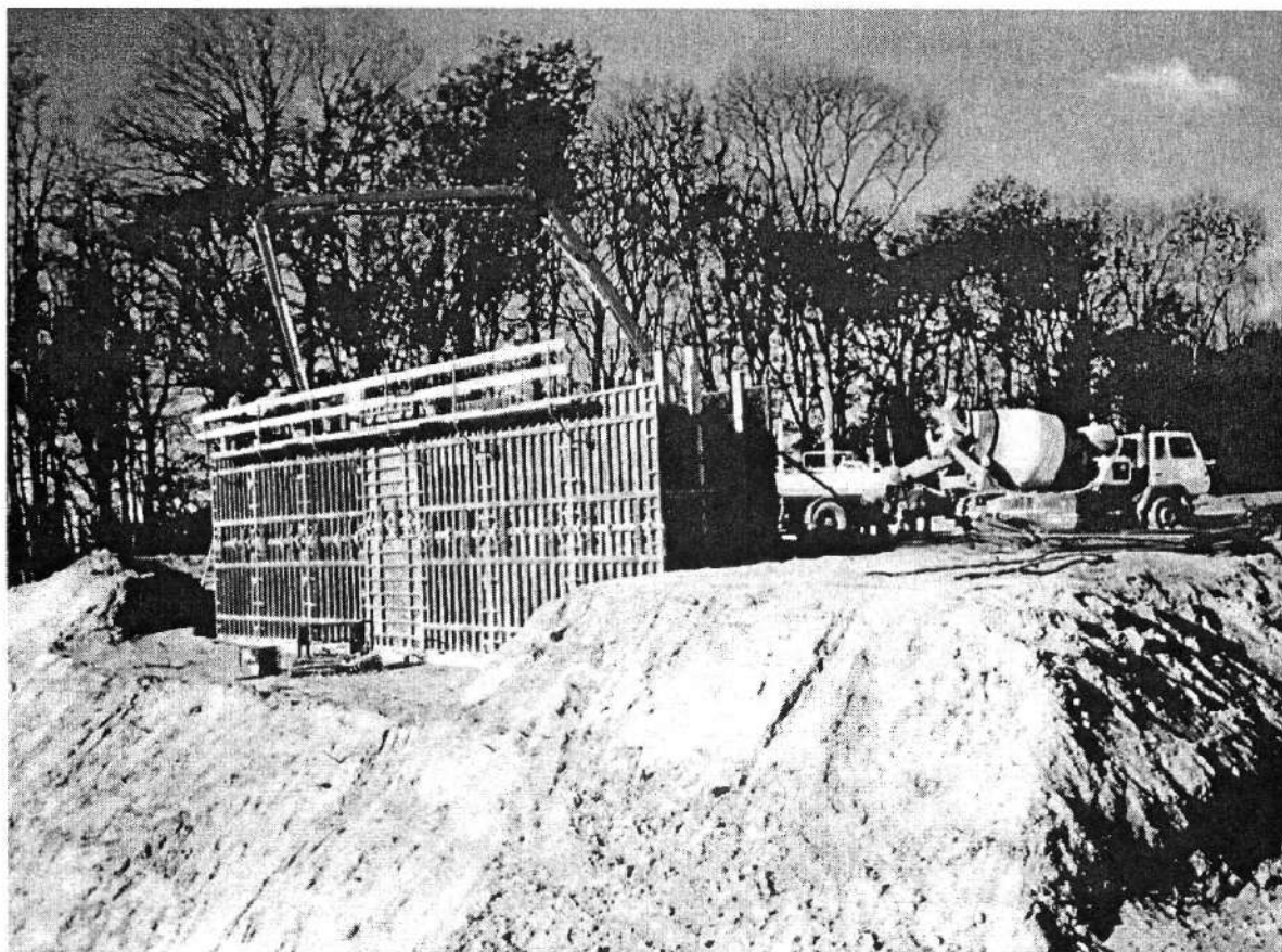
Hídfő betonozása (1. kép)
