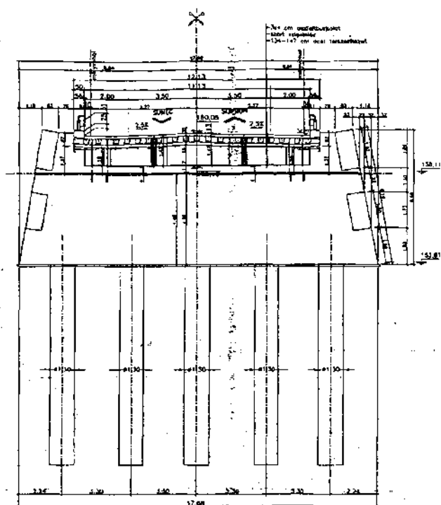
MEDER TÁMASZ (D) KERESZTMETSZET M1:100 (62+775,25 SZ.)
